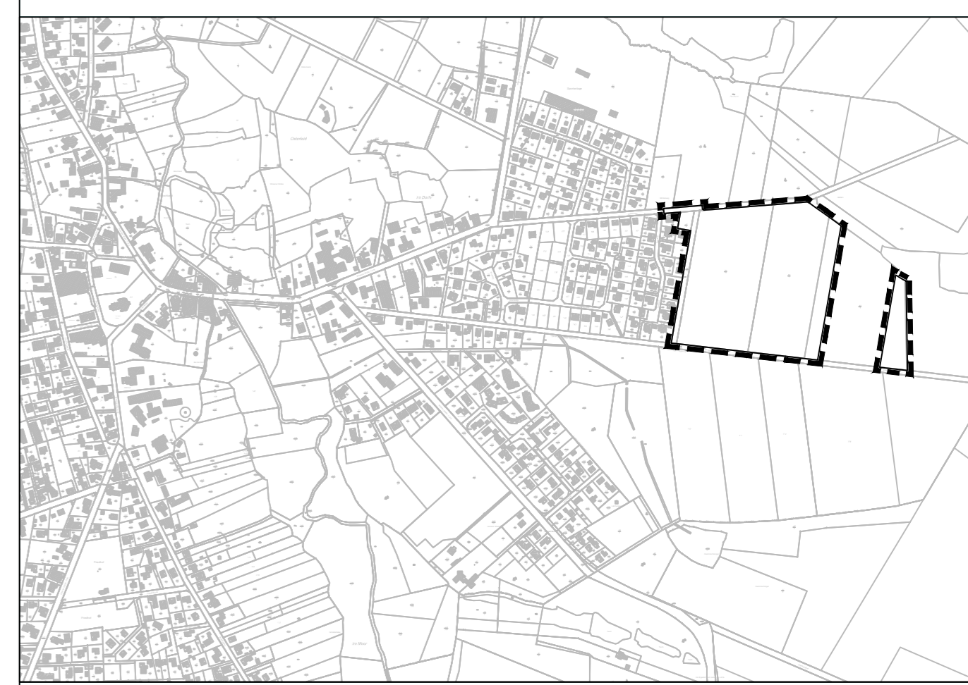
Übersichtsplan, M 1:10.000
